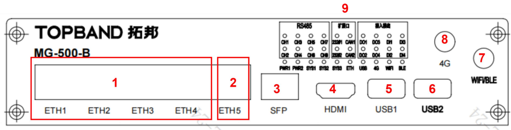
图 2 前面板示意图
